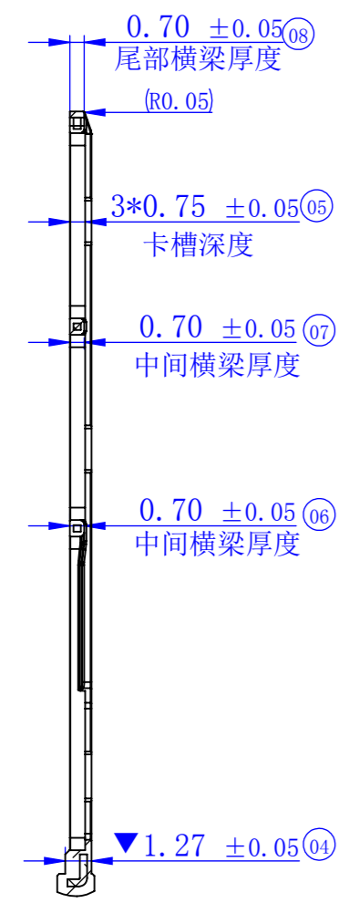
剖面 AD-AD 比例 3 : 1
